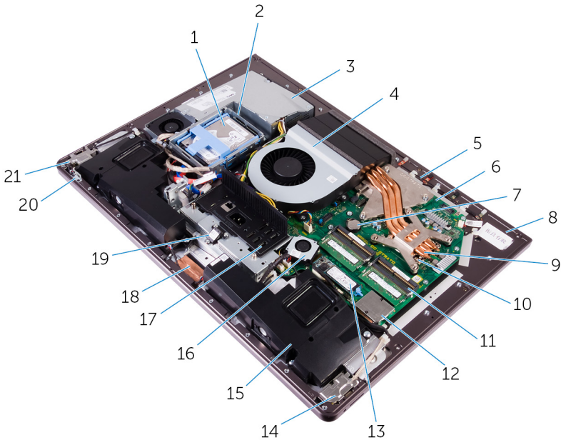
Figur 2. : Innsiden av datamaskinen (uten berørings skjerm)
